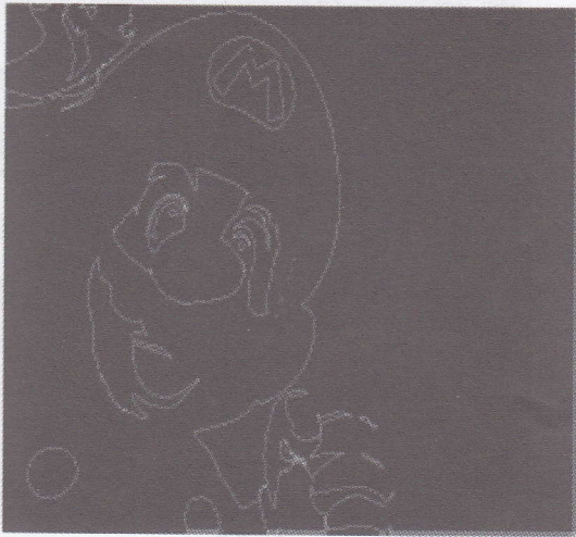
Gambar. 17. Remove
