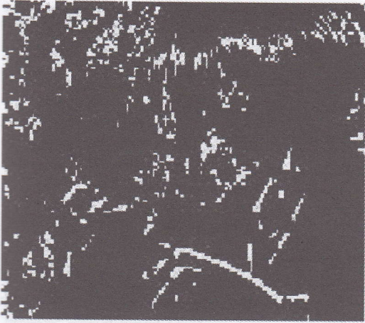
Gambar. 27. Top Hat
