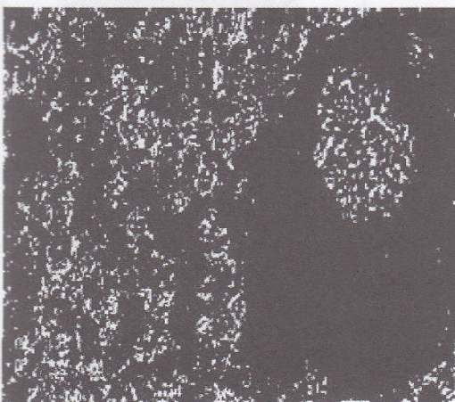
Gambar. 55. Top Hat
