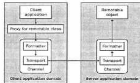
Gambar 2. Arsitektur .NET Remoting
