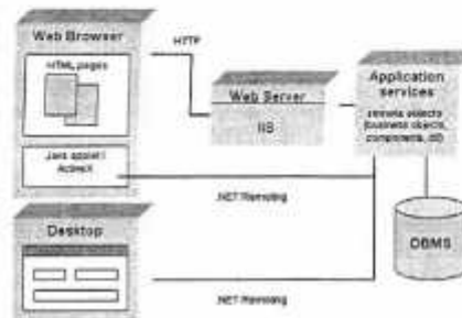
Gambar 3. Arsitektur Sistem
